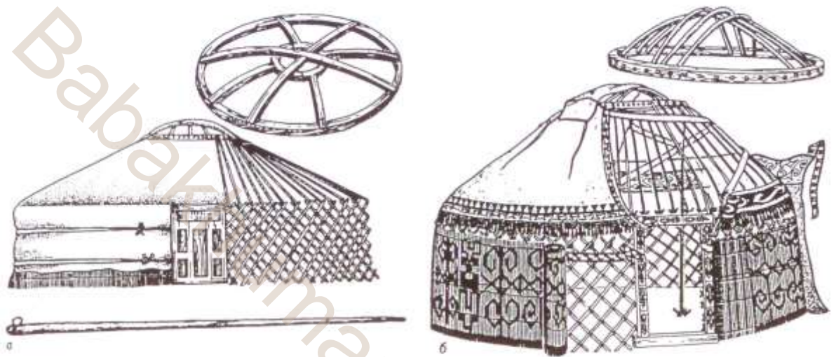
Рис. 7. Конструктивные особенности деревянного остова юрты: а – монголов; б – северных киргизов
